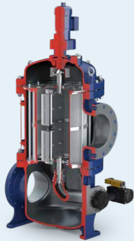
Feinsiebzylindereinsatz
