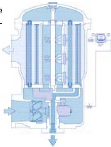
BOLLFILTER 自清滤器 型号 6.46
