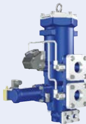
BOLLFILTER 自清滤器型号 6.21/6.22
